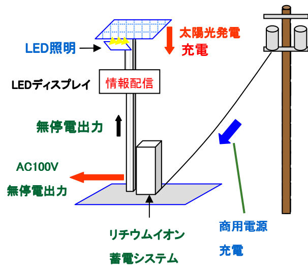
「多機能防災システム」イメージ図
