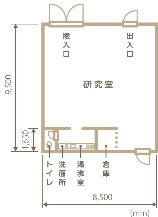
間取り
